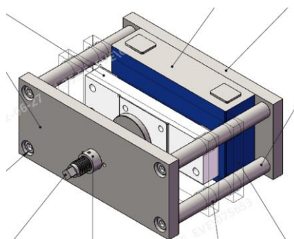
膨胀力夹具安装图
