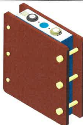
Fig. 4 Side view of cell shaft 图 4 电池轴侧图
