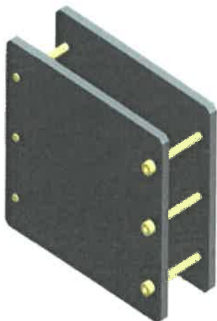
Fig. 1 Schematic diagram of cell clamp 图 1 电池夹具示意图
