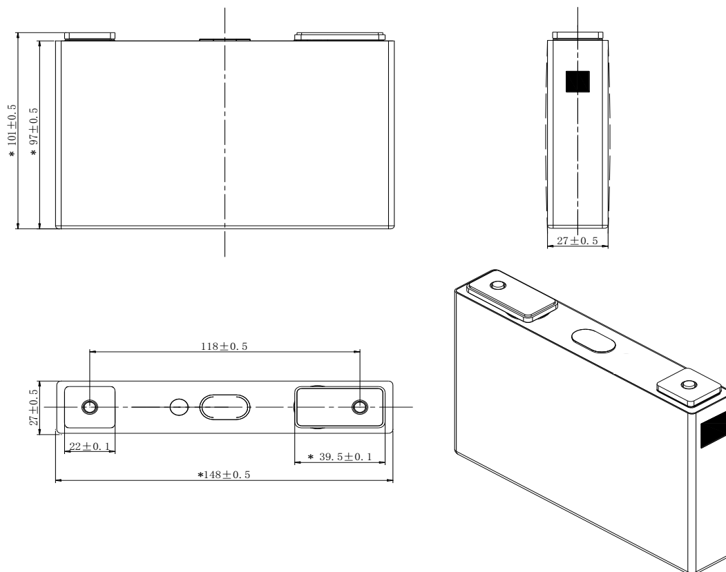
图 A.1 电池尺寸图
