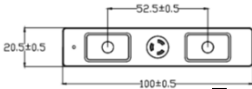
电芯盖板尺寸
