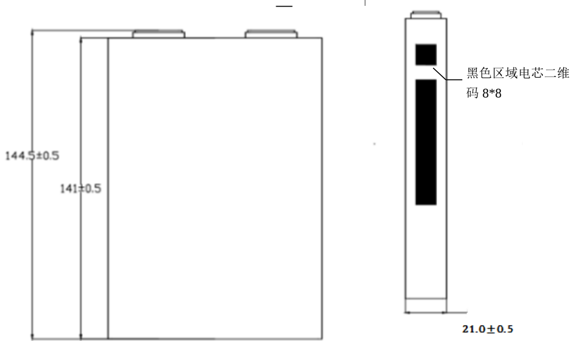
电芯整体尺寸
