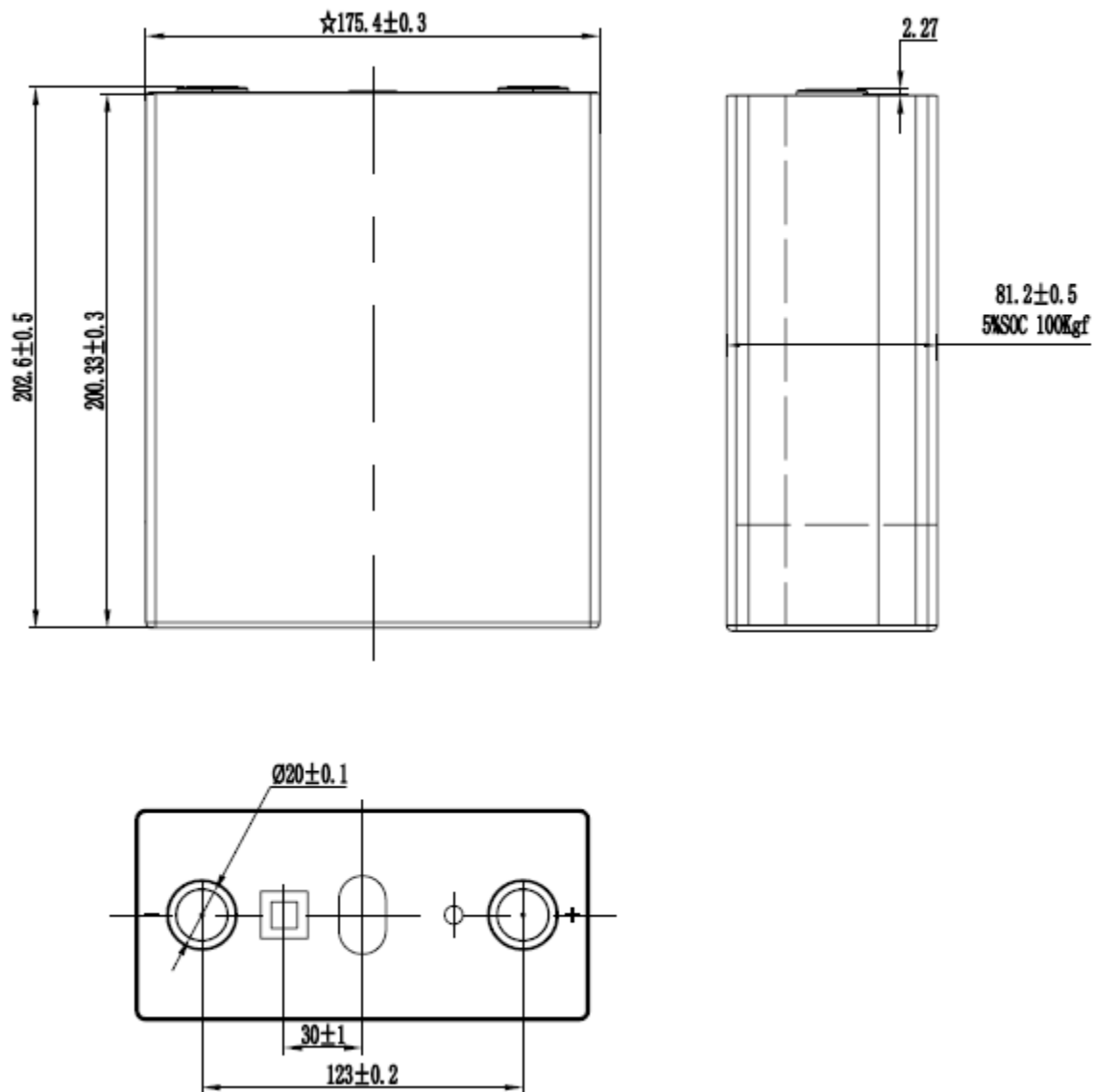
电芯整体尺寸
