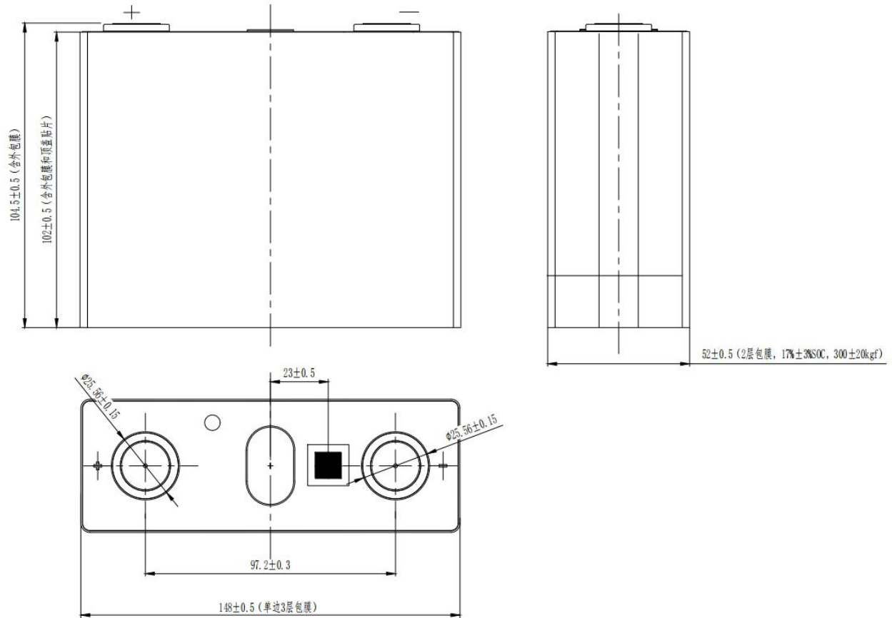
电芯尺寸 Cell Dimension
