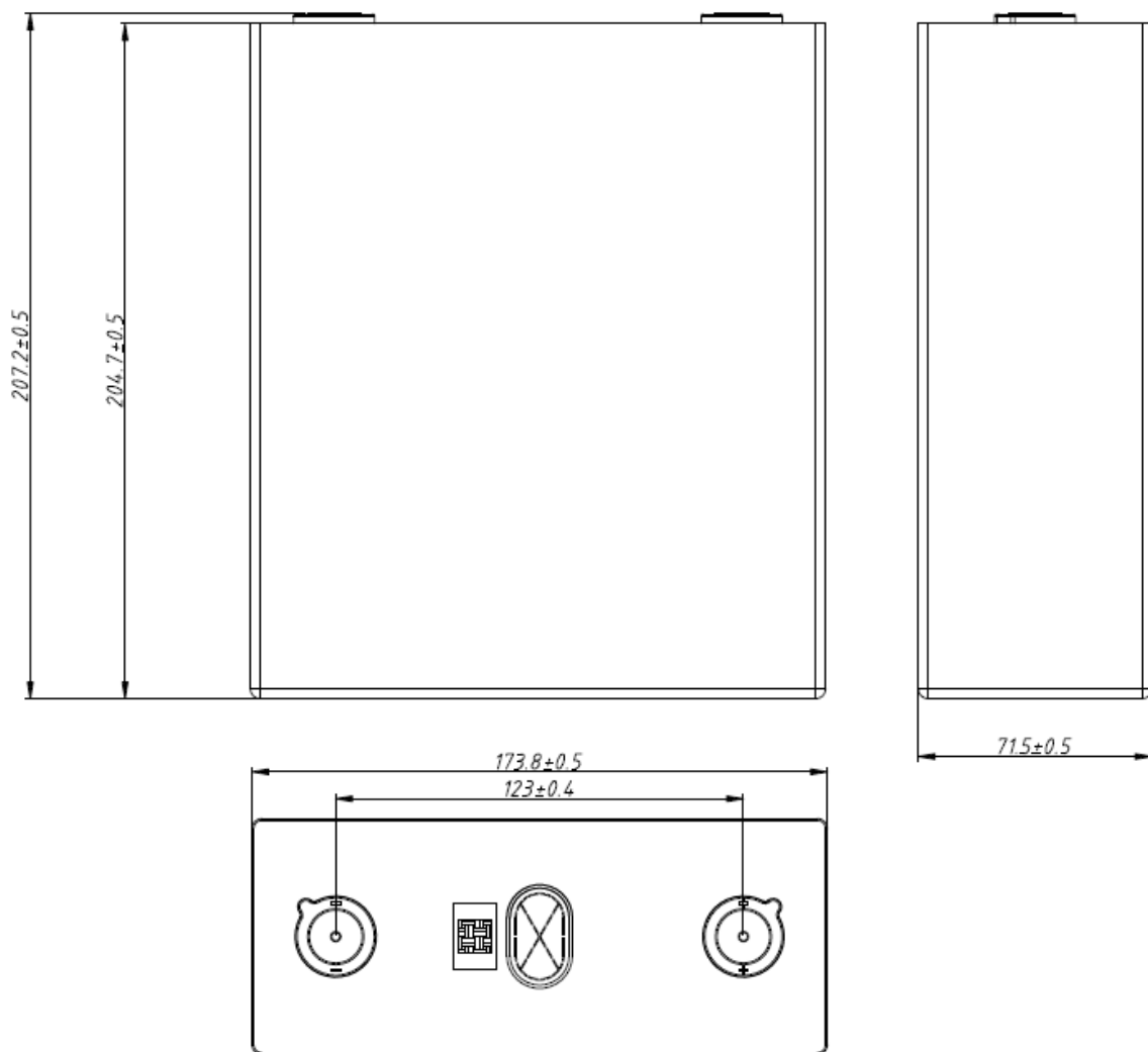
图 1 电池简易外形图（含蓝膜）
